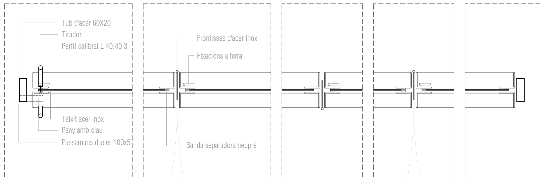
SECCIÓ HORITZONTAL E.1/5
