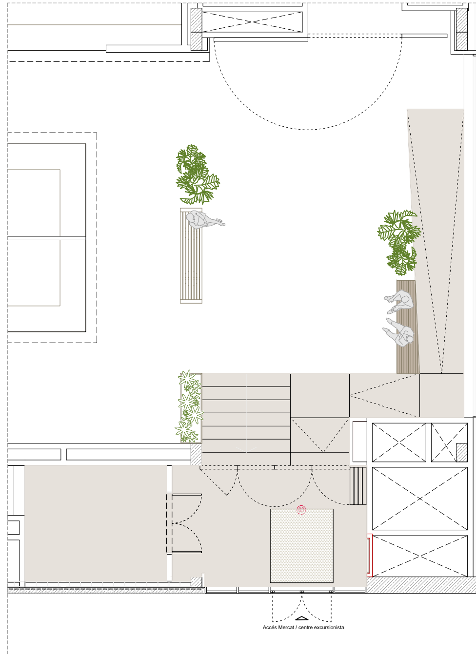
Vestíbul muntanya | Proposta
