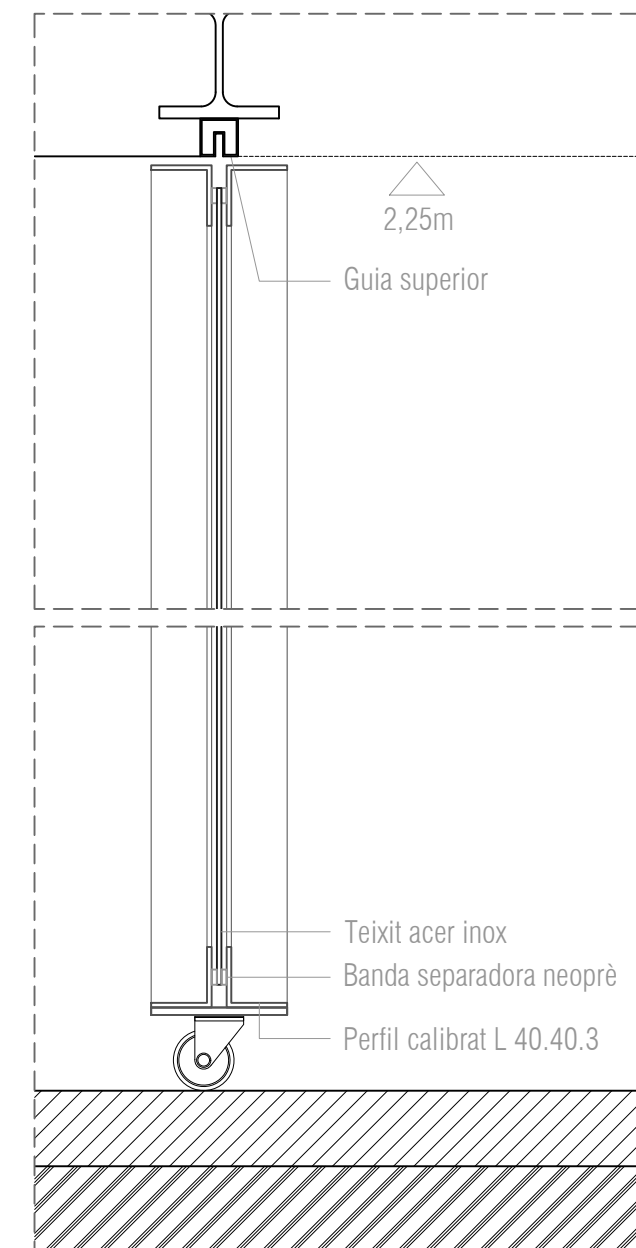
SECCIÓ VERTICAL E.1/5
